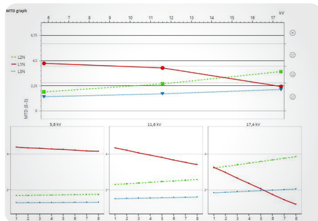
Visualización de una medición del factor de disipación en el informe de ensayo ↑
